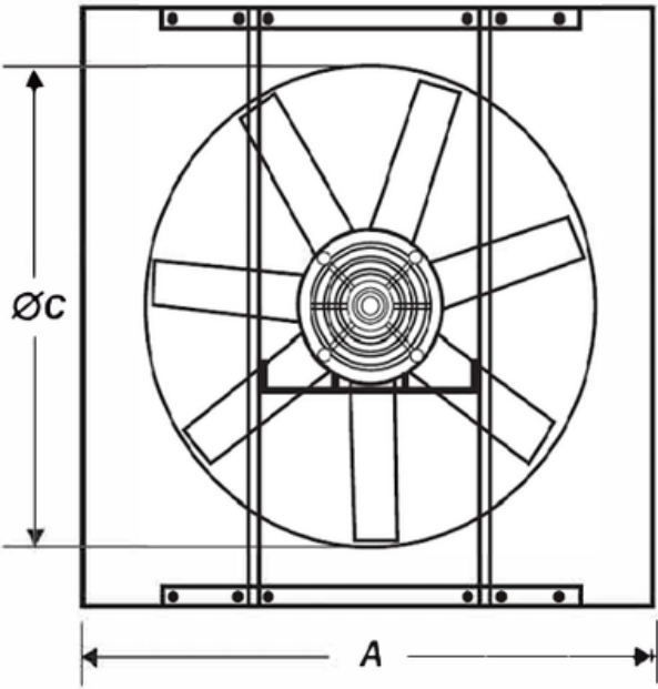
VISTA POSTERIOR (BACK VIEW)
